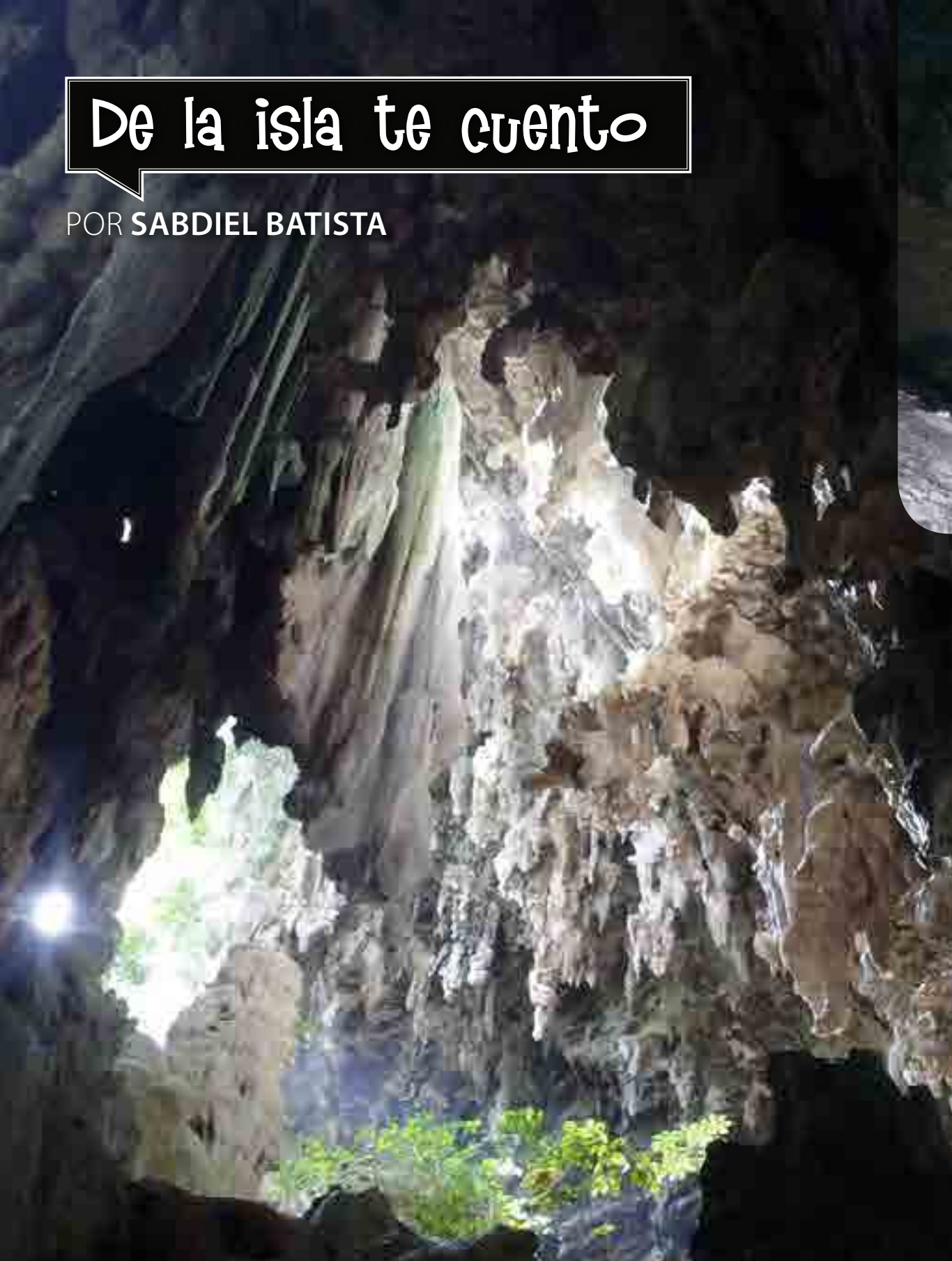
En la Cueva Martín Infierno se puede observar la estalagmita más alta del mundo.
